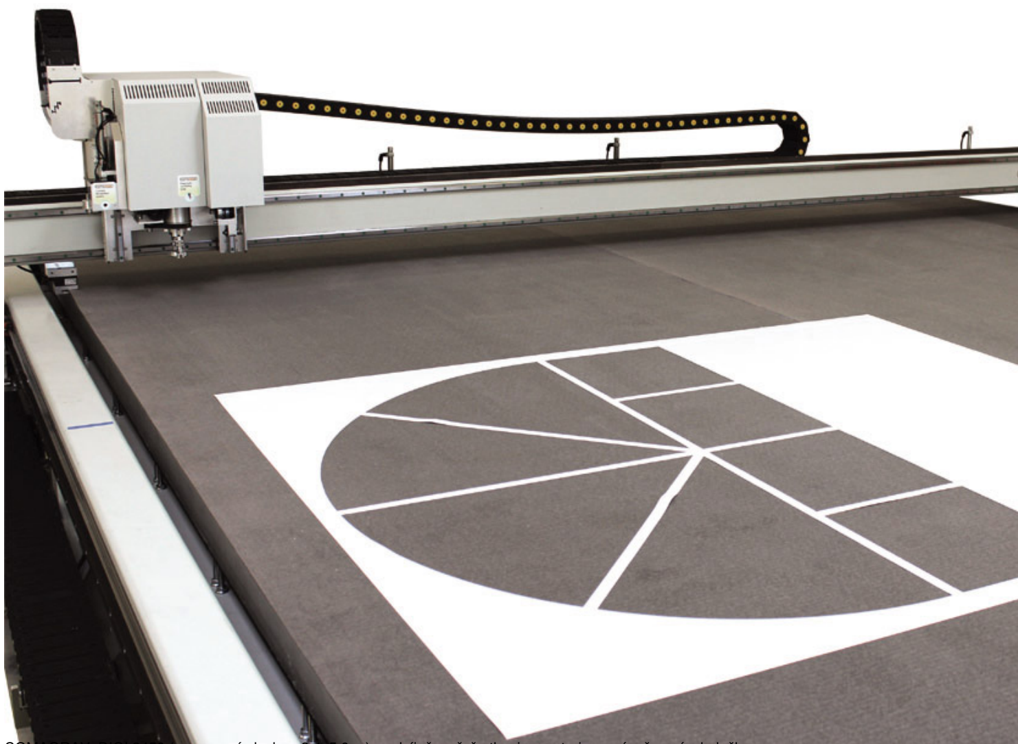
COMAGRAV DIGI 3450 (s pracovní plochou 3,4x5,0 m) s odvíječem řeže tkaninu motorizovaným řezacím kolečkem
